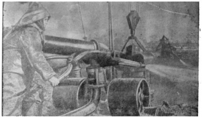
Добыча торфа гидромонитором на торфопредприятии «Лазия» (Ленинградская область). Фото Н. Караева. Прессклише ТАСС
