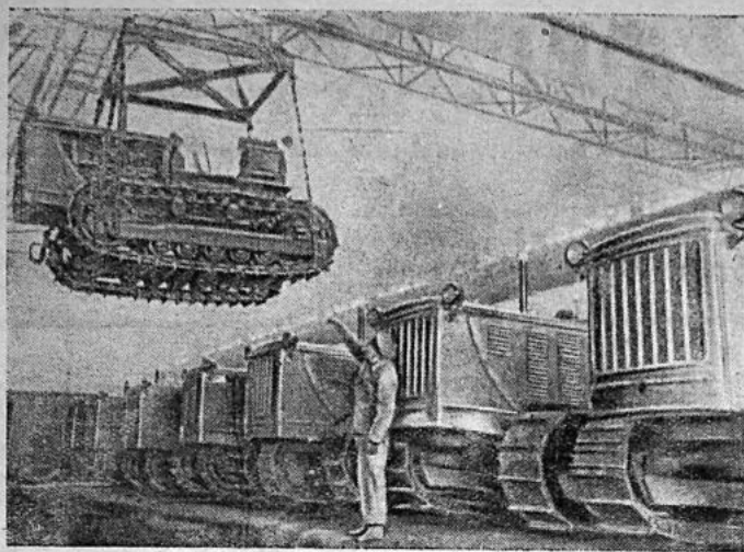
Челябинск. С конвейера Кировского завода на Урале сходят мощные гусеничные тракторы «С-80». На снимке: тракторы «С-80» перед погрузкой на железнодорожные платформы. Фото П. Шучкина. Прессклише ТАСС.
