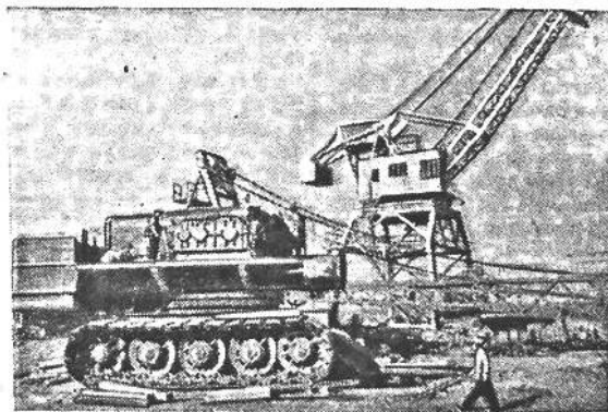
На монтажных площадках строительства Тахна-Ташского гидроузла идет сборка семикубовых электрических экскаваторов, предназначенных для рытья котлованов.
