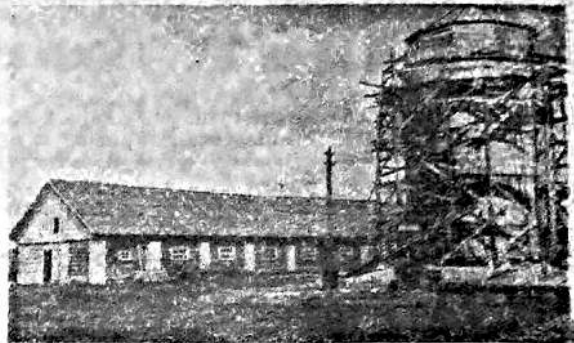
В колхозе им. Молотова сейчас завершается строительство сборной деревянной башни для силосования, емкостью на 150 тонн. Фото Е. Давыдовой.
