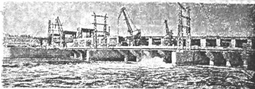
Строители Камского гидроузла подводят первые итоги своего труда. Уже дан в эксплуатацию судоходный шлюз. В сентябре две турбины гидроэлектростанции дали промышленный ток. Сейчас навешиваются провода высоковольтной линии Молотов—Свердловск. На снимке: общий вид водосливной плотины Камской гидроэлектростанции.
