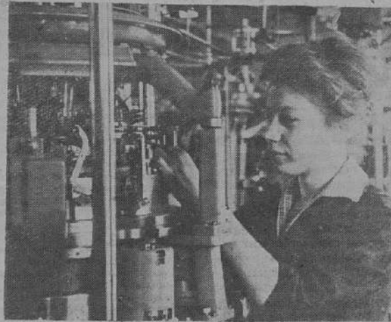
В вязальном цехе трикотажной фабрики имени Розы Люксембург уже работают на полную мощность несколько недавно смонтированных новых круглофанговых машин. На нашем снимке молодая работница Тамара Метель. Одной из первых на фабрике она освоила работу на новой технике. Фото Н. Кривенко.
