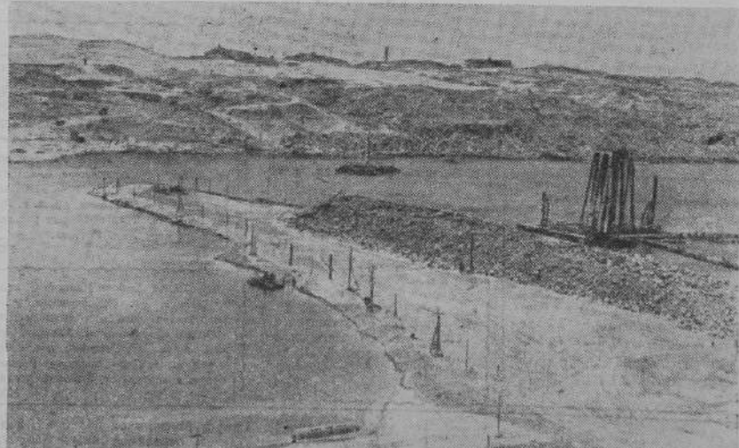
Асуан (Объединенная Арабская Республика). Последние дни перед перекрытием Нила. На снимке: вид на проран с правого берега.
