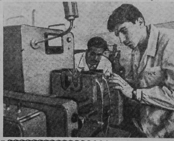
АРМЯНСКАЯ ССР. На Кировоаканском заводе прецизионных станков начато серийное производство станка модели 9710 для балансировки вращающихся деталей двигателей. Он спроектирован Московским экспериментальным научно-исследовательским институтом металлорежущих станков. На снимке: мастер балансировочного участка Т. Овакмян (слева) и наладчик М. Тертерян у нового станка.
