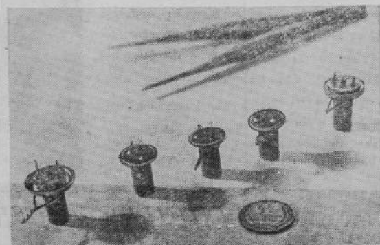
На снимке: полупроводниковые квантовые генераторы (лазеры), созданные в физическом институте Академии наук СССР, имени П. Н. Лебедева.
