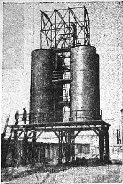
На Загорской реализации базе хлебных продуктов идет монтаж склада для белгарики складирования импортной муки (компонент комбикорма). На металлическое основание установлены четыре цилиндрических бункера емкостью по 30 тонн каждый. Строительство ведет Московское областное управление хлебопродуктов и комбикормовой промышленности (начальник участка И. Зорин). Монтажные работы будут закончены в середине года.
