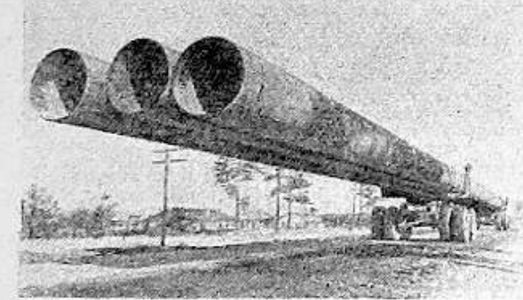
На строительстве газопровода Шелбино-Брянск применяется новая техника — землеройные машины, отвальные машины, бульдозеры. Доставка 36-метровых труб на участке Брянск-Кромь осуществляется плетевозом. На снимке: транспортировка труб плетевозом. Фотография ТАСС.
