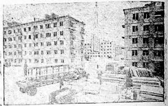
Москва. В Верхних Мещанинах, где развернулось большое жилищное строительство, дома монтируются из железобетонных блоков непосредственно на площадке. Таким способом пятиэтажный жилой дом монтируется и отделывается за 56 дней. На снимке из обзора по участку строительства крупнопанельных домов в Верхних Мещанинах.
